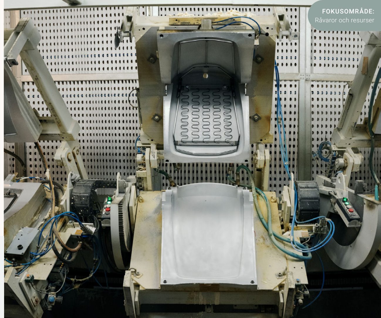
Skumgjutning av stolar i vår fabrik i Skillingaryd.
